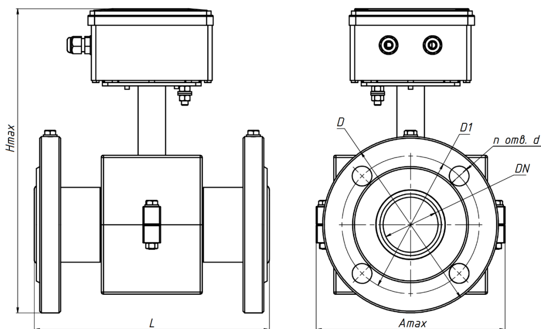
Рисунок Б.6 Габаритные и установочные размеры ПРП
