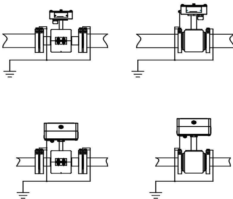
Рисунок 6.6 Заземление расходомера
