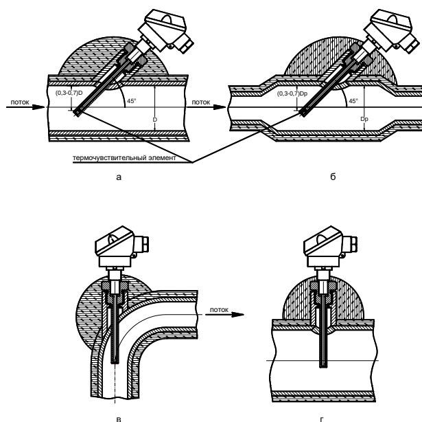
Рисунок 6.8 Рекомендуемые варианты установки термopеобpазователей на трубопроводе
